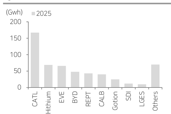
Fig. 24: 2025년 기업별 ESS 출하량
