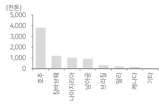
Fig. 36: 중국 국가별 스포듀민 수입량(2025)
