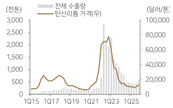
Focus Chart 4 칠레 탄산리튬 수출량 및 리튬가격 추이
