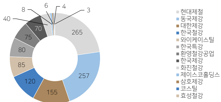
Fig. 49: 한국 철근 생산능력 현황
