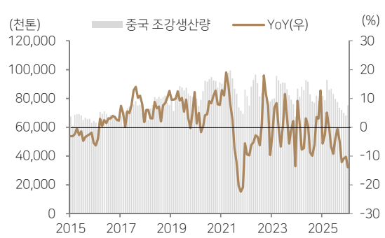
Fig. 19: 중국 조강생산량 추이(월별)
