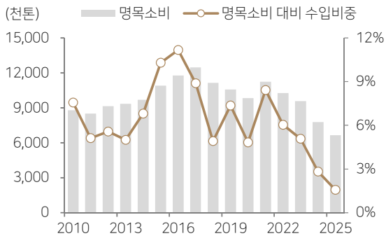
Fig. 5: 철근 명목소비 및 수입비중 추이
